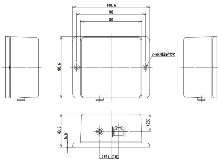
図: HP-400f(LAN)外形図
